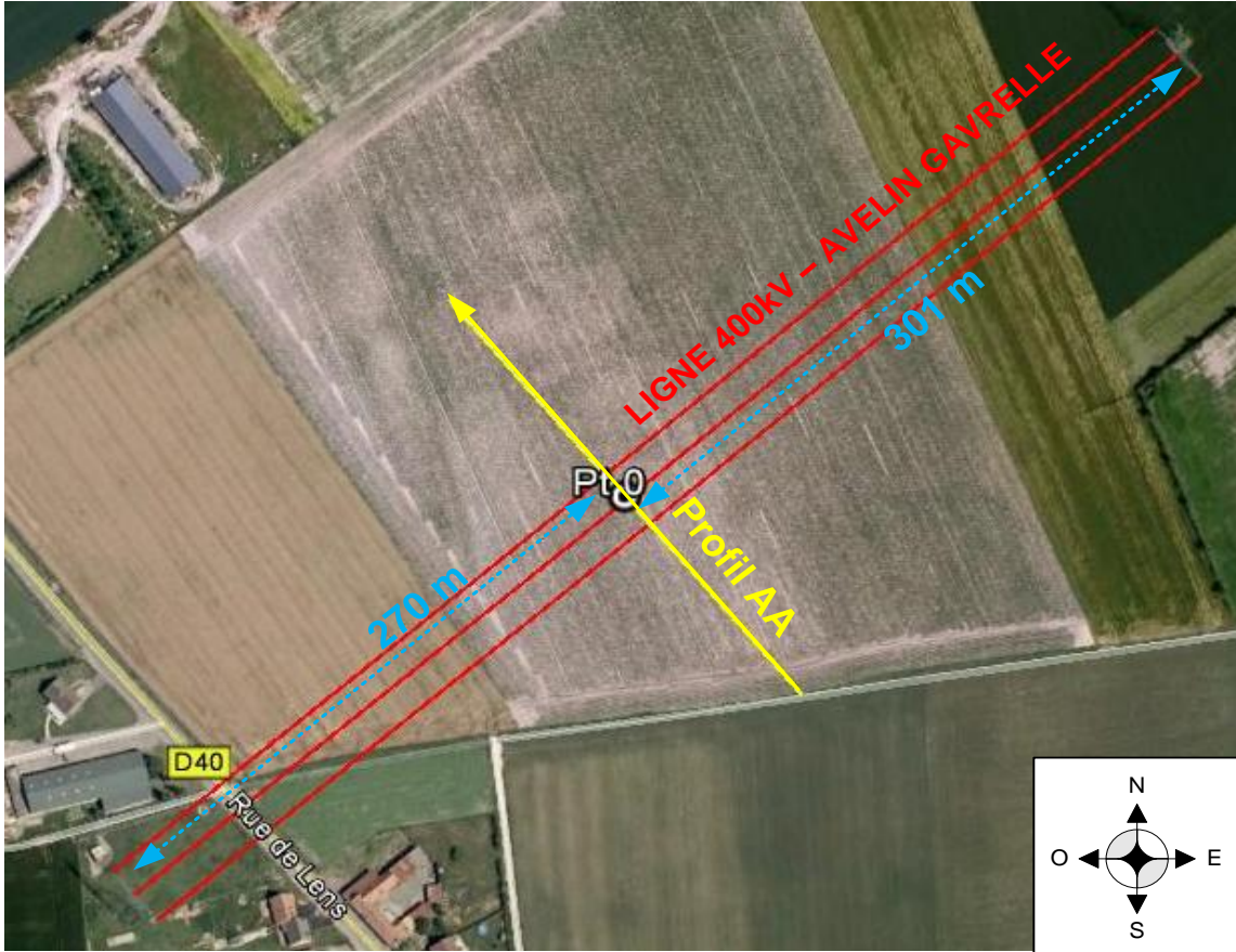
Pylône 368
